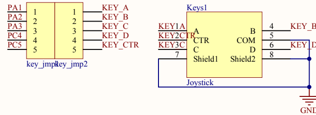
JOYSTICK
