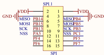
SPI1
