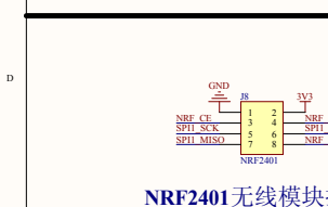
NRF2401无线模块接口
