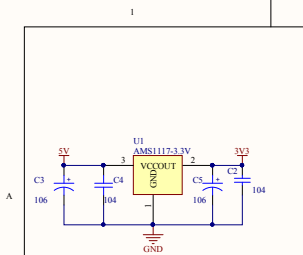
系统稳压供电
