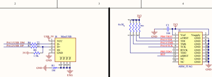
STM32-USB Slave接口
