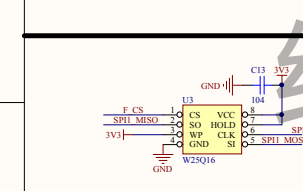
FLASH--W25Q16
