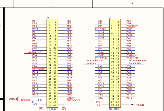
系统可用I/O外引接口
