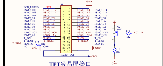
TFT液晶屏接口
