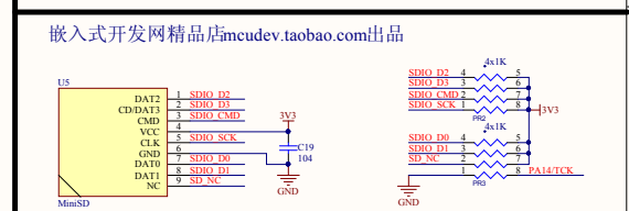
TF-SD存储卡座
