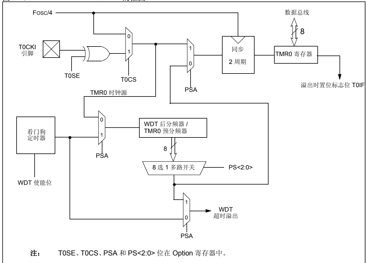
图 6-1: TIMER0/WDT 的框图
