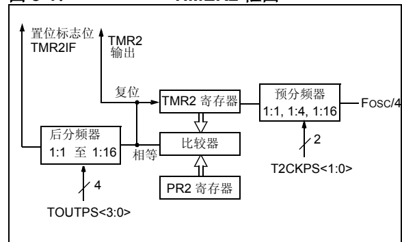
图 8-1: TIMER2 框图
