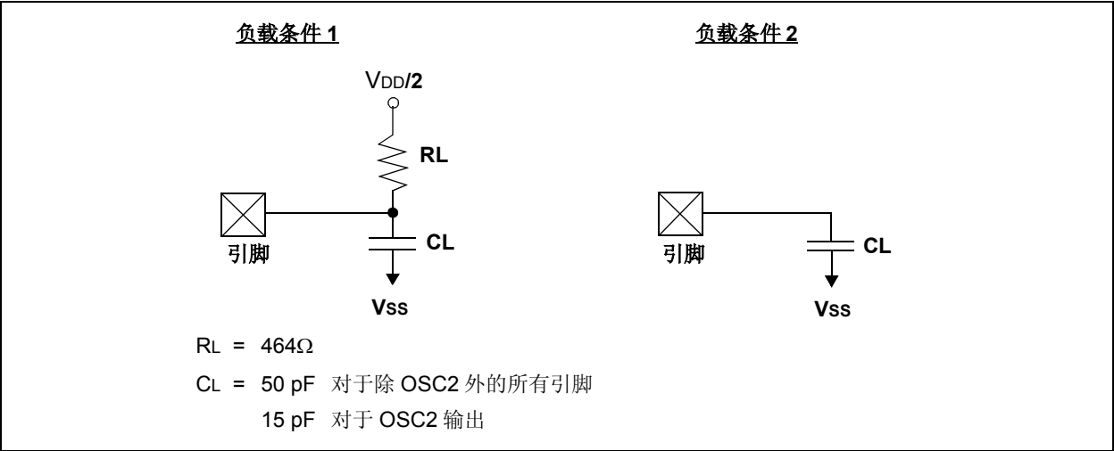
图 17-3： 负载条件
