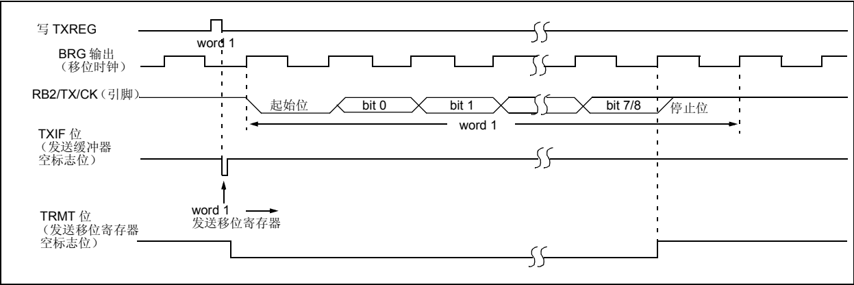
图 12-2: 异步发送
