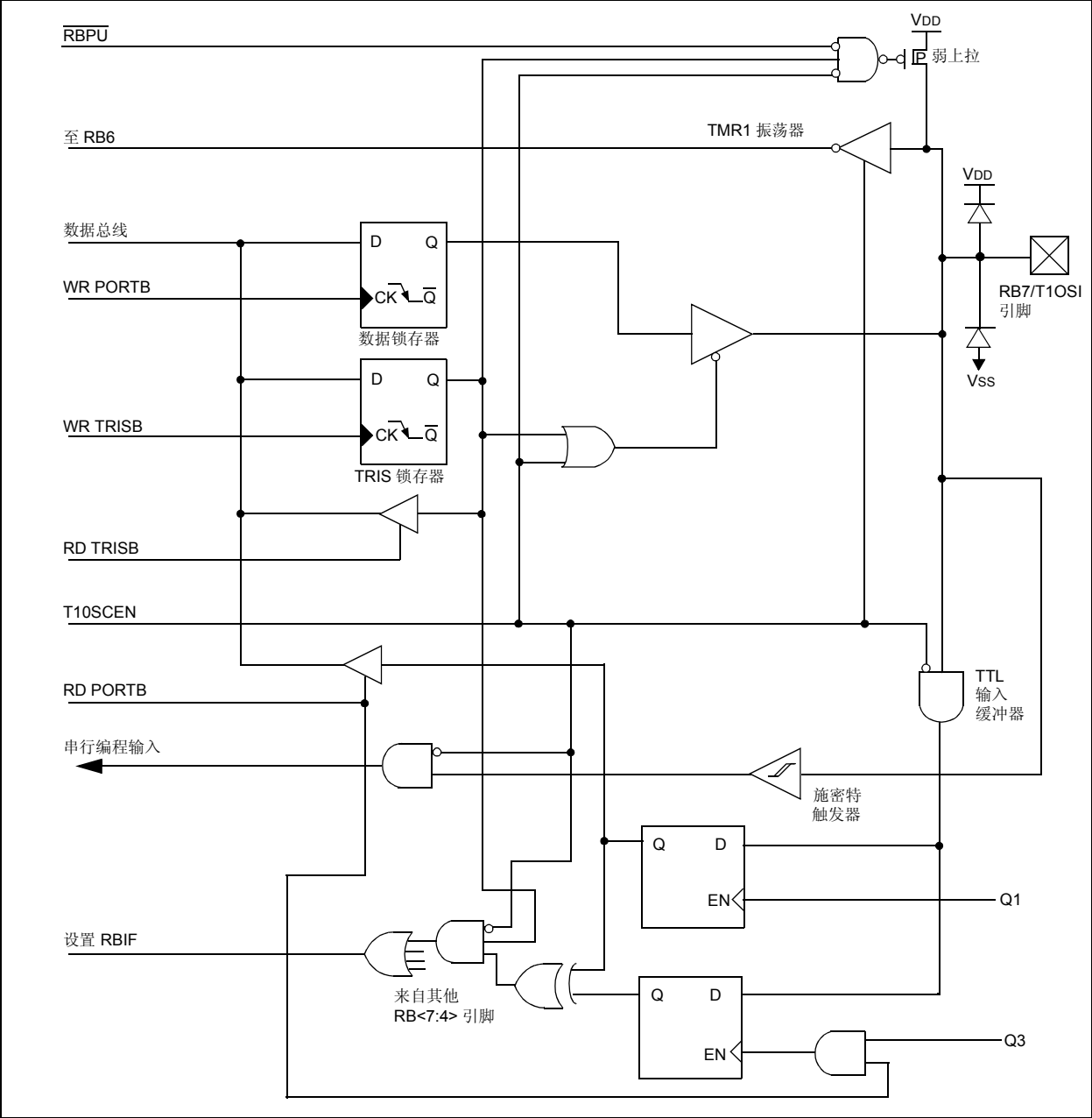
图 5-15: RB7/T10SI 引脚框图
