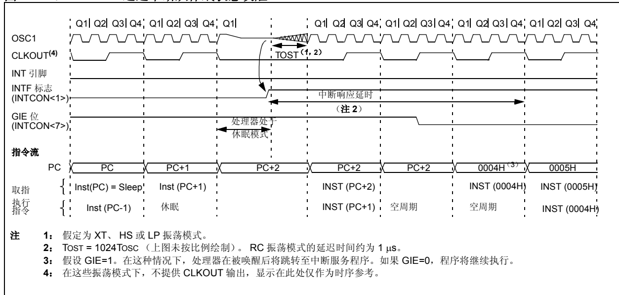
图 14-17: 通过中断从休眠状态唤醒
