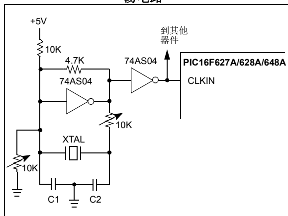
图 14-2: 外部并联谐振器 / 晶振的振荡电路
