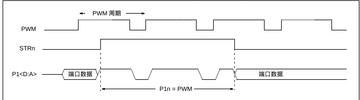
图 11-19 : 指令结束时发生的转向事件的示例 (STRSYNC = 0)
