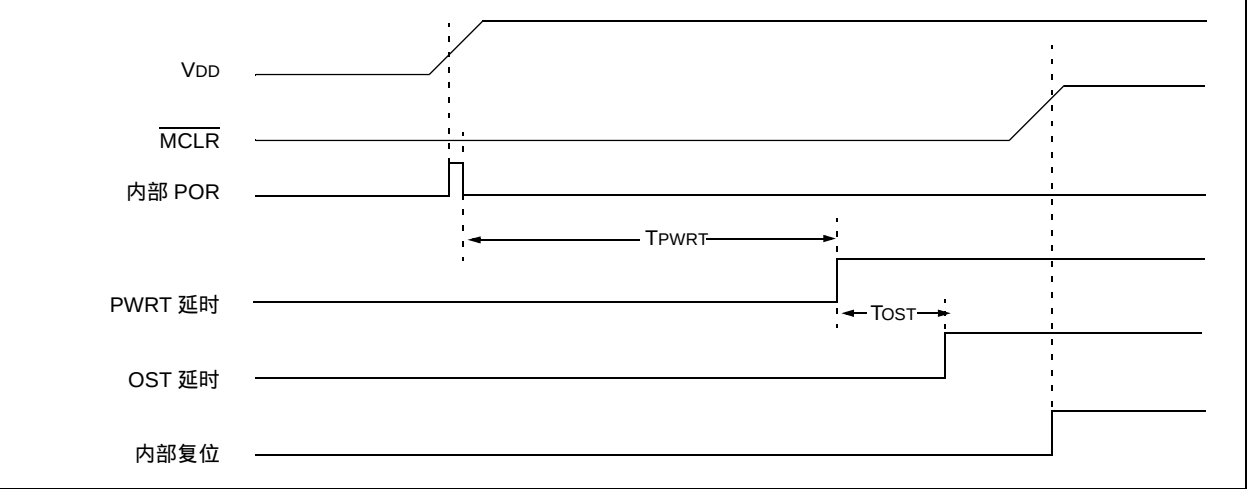
图 14-5 : 上电时的延时时序 (MCLR 延时) : 情形 2
