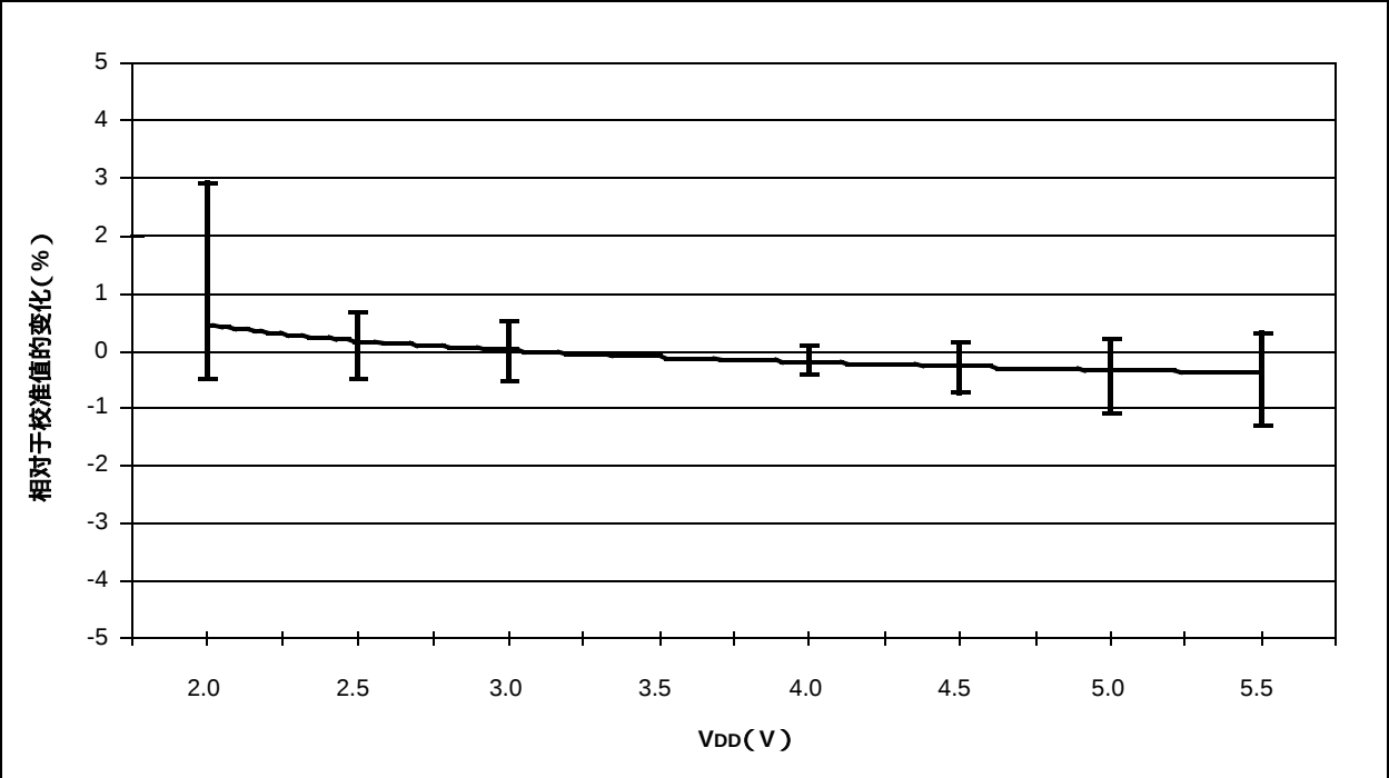
图 18-35 : 典型 HFINTOSC 频率变化 - VDD 关系曲线 (25°C)
