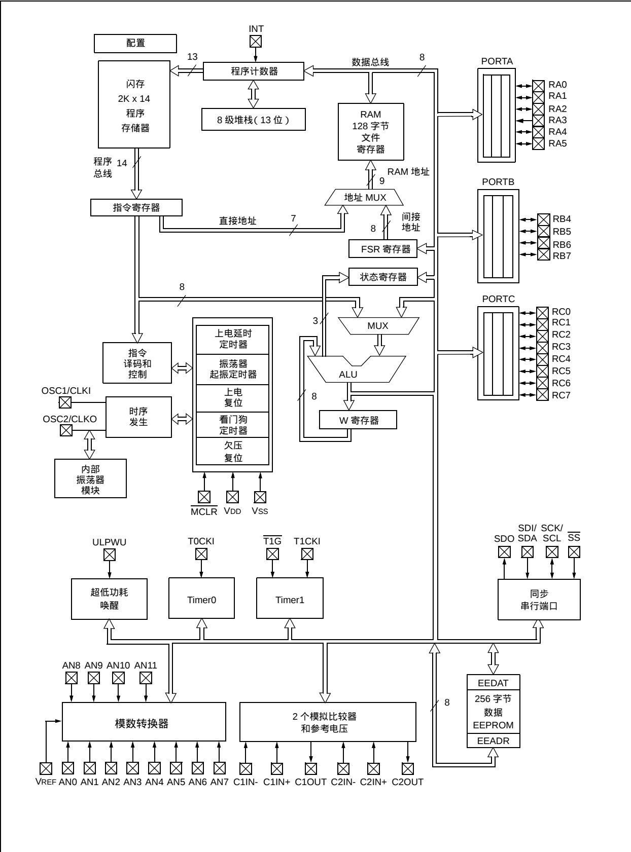
图 1-2 : PIC16F677 框图
