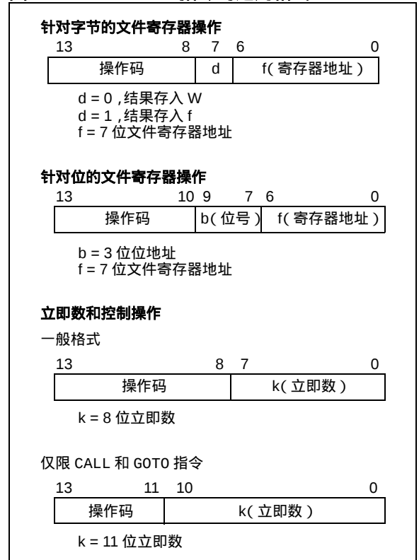
图 15-1：指令的通用格式
