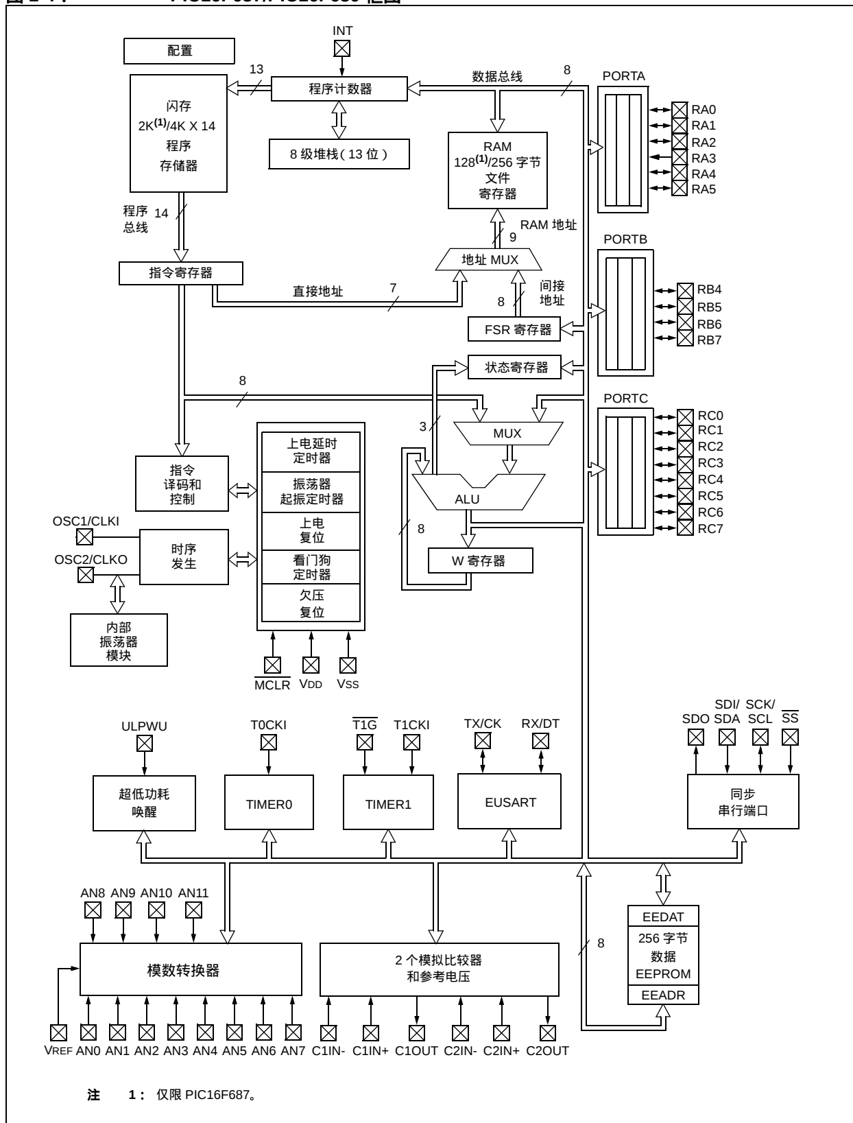
图 1-4 : PIC16F687/PIC16F689 框图
