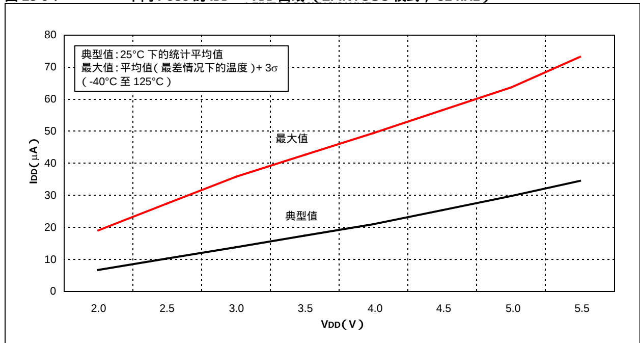
图 18-9：不同 FOSC 的 I_{DD} - V_{DD} 曲线（LFINTOSC 模式，31 kHz）
