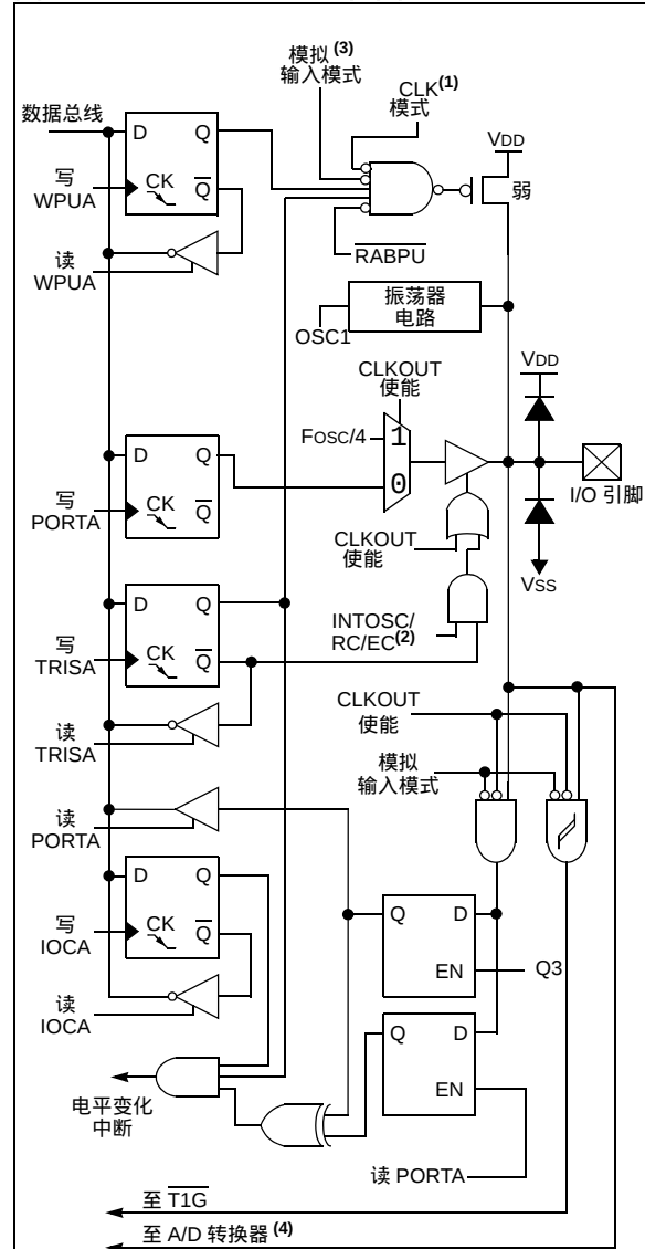
图 4-5： RA4 框图
