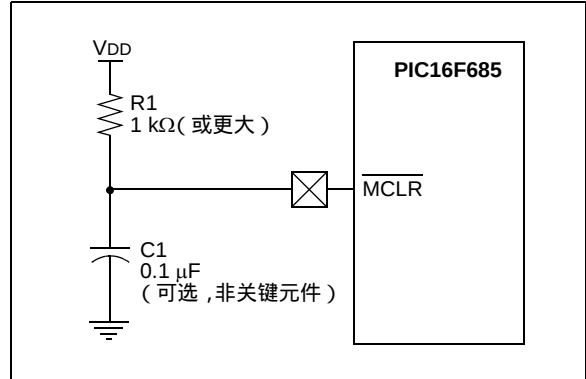
图 14-2： 建议的 \overline{\text{MCLR}} 电路
