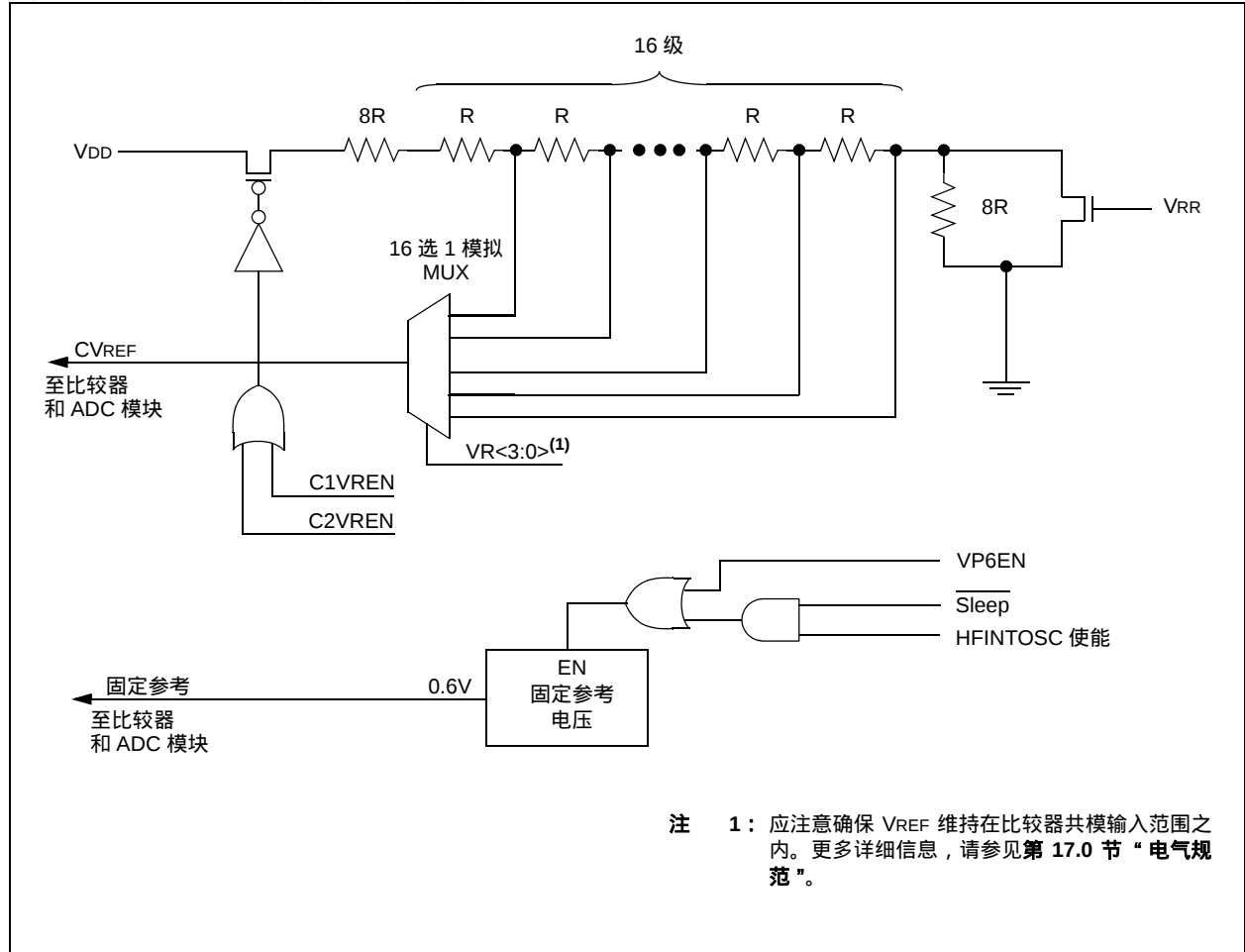
图 8-8： 比较器参考电压框图
