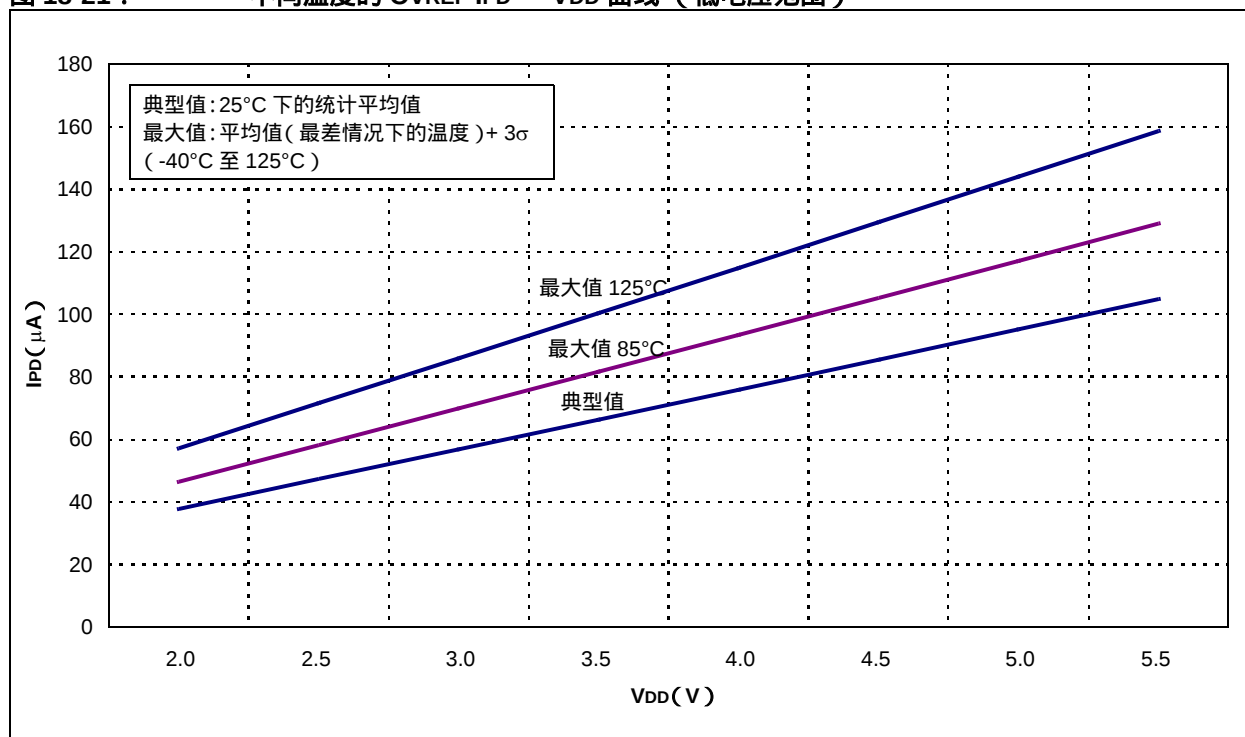
图 18-21 : 不同温度的 CVREF IPD - VDD 曲线 (低电压范围)
