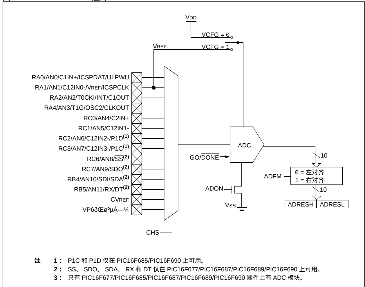
图 9-1： ADC 框图
