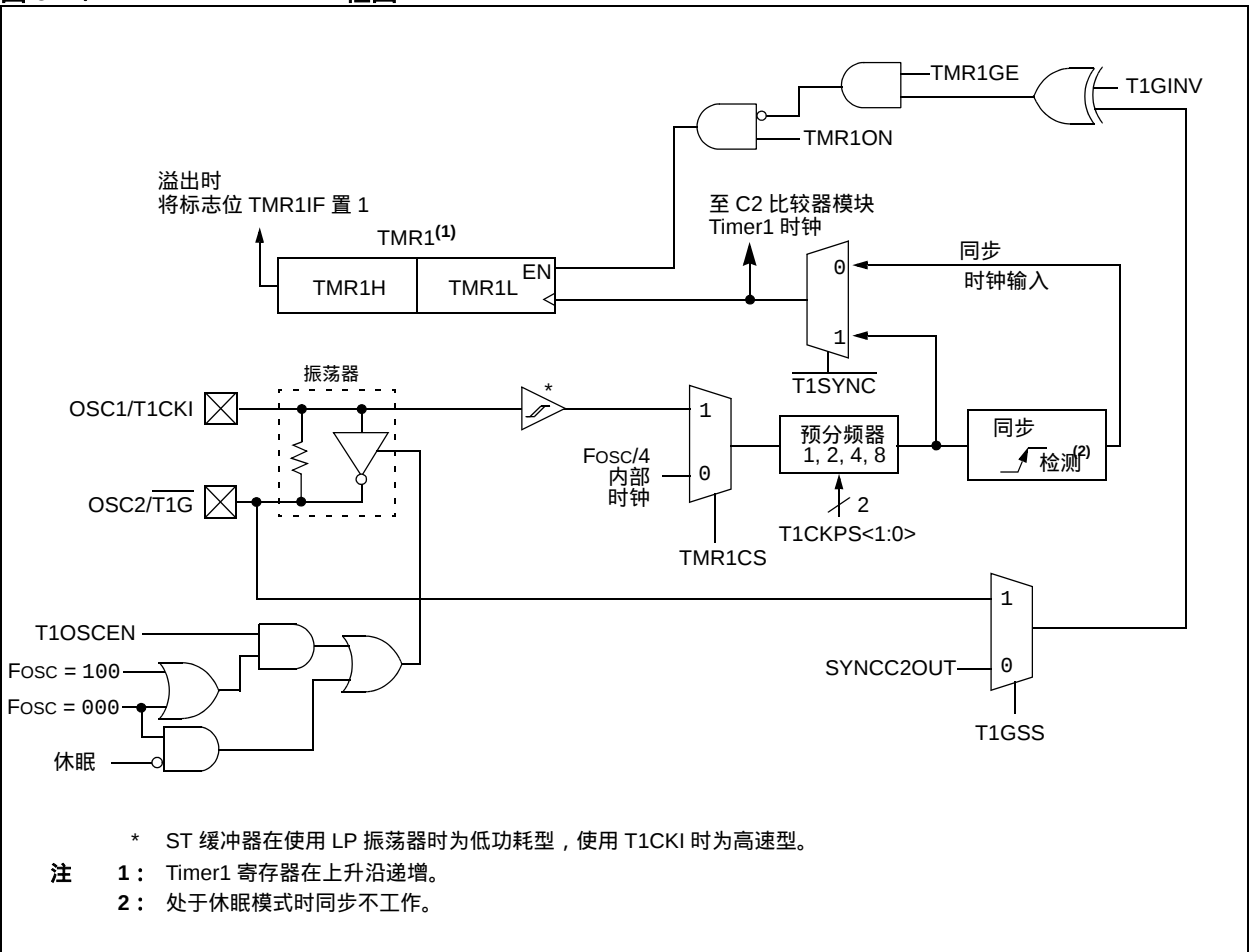
图 6-1：TIMER1 框图
