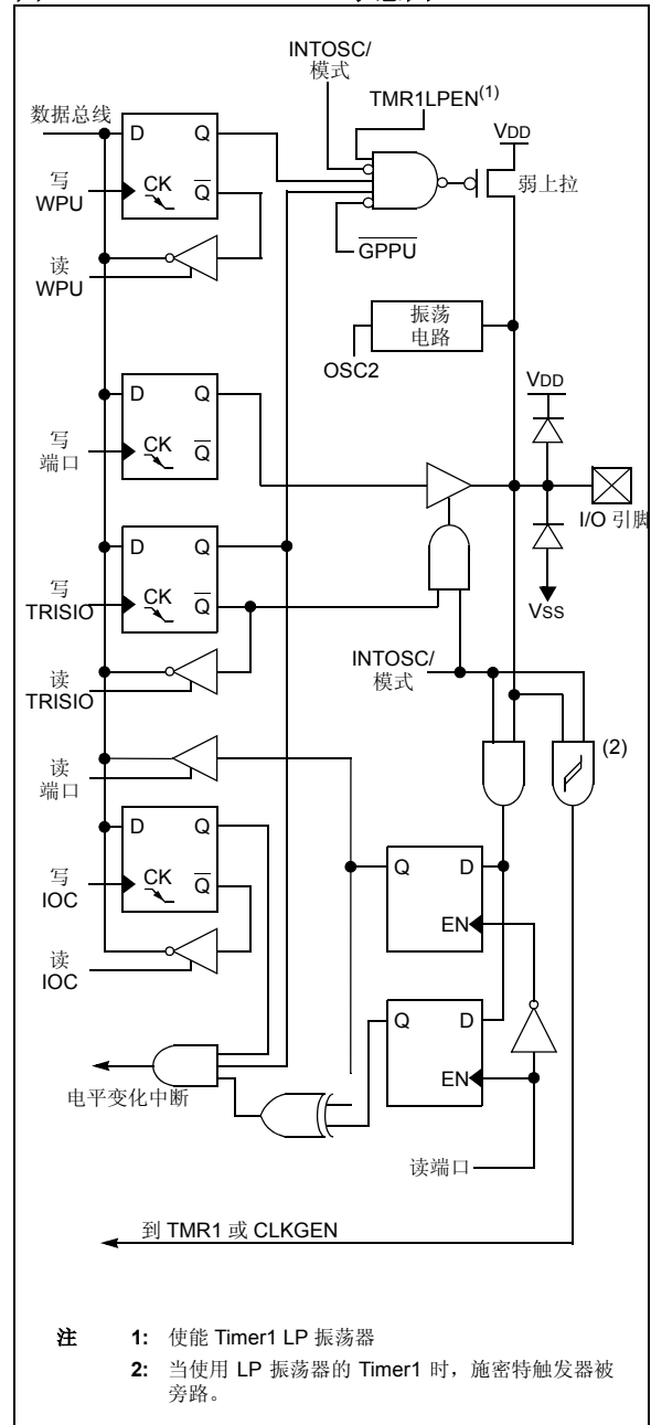
图 3-5: GP5 示意图
