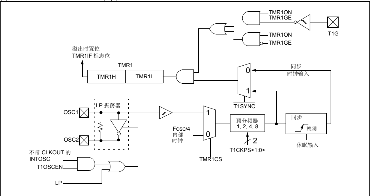
图 5-1: TIMER1 框图
