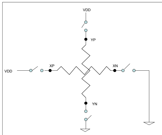
图 6-44 : 4-wire 触控面板原理
