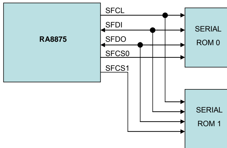
图 6-35 : RA8875 串行式 Flash/ROM 系统
