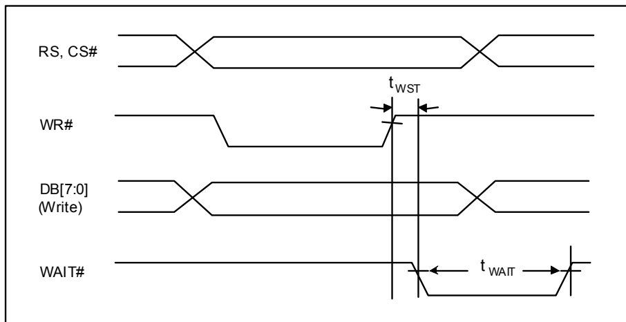
图 6-29 : WAIT# 时序图
