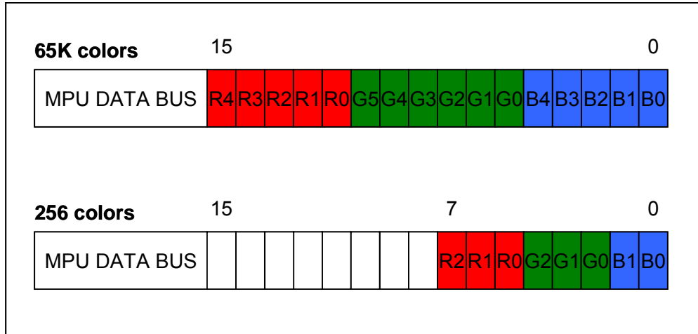
图 6-30 : MCU 16-bit 时 Data Bus 所对应到的 RGB 数据
