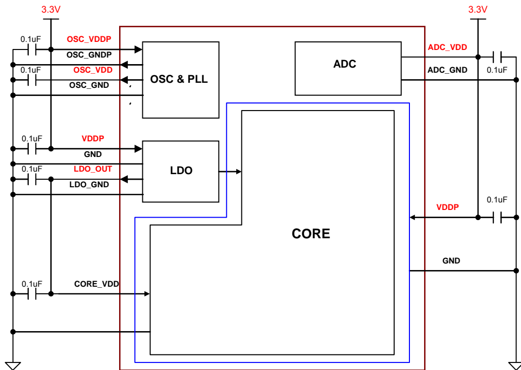
图 6-51 : RA8875 的电源接法
