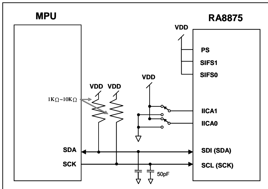
图 6-21 : IIC 的 MCU 界面图
