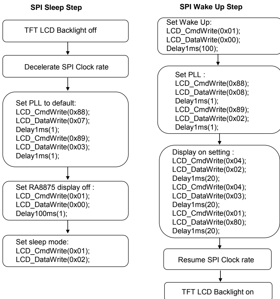
圖6-20 : SPI 睡眠/喚醒
