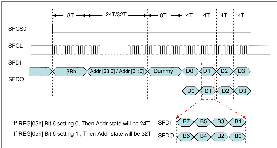
图 6-39 : 双倍模式 - 0 读取
