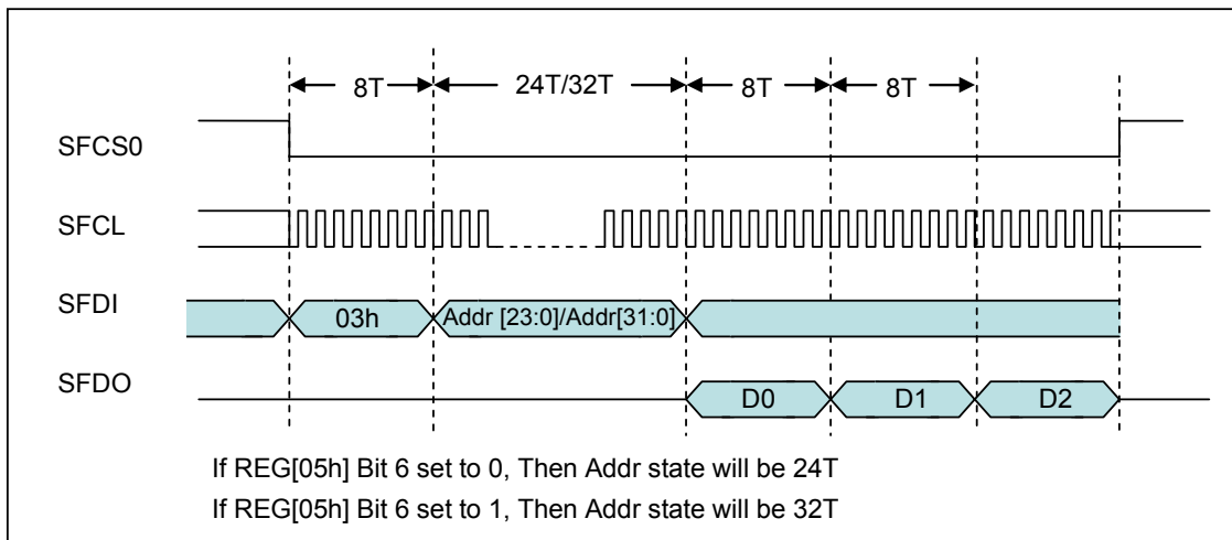
图 6-37 : 4-BUS (正常) 读取
