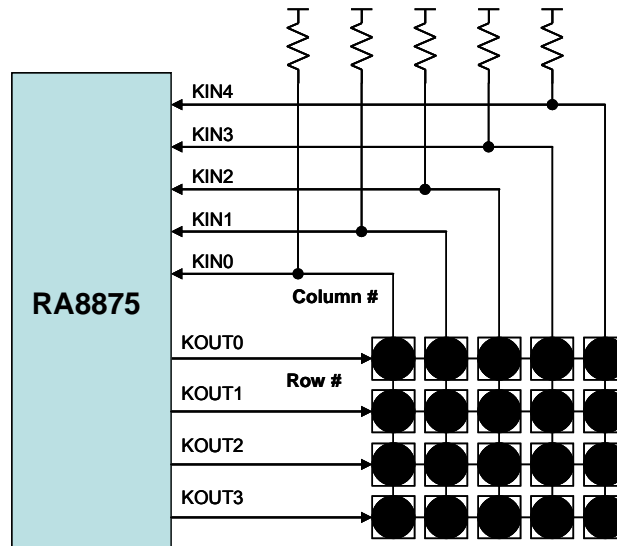
图 6-46 : 4x5 键盘的基本应用电路
