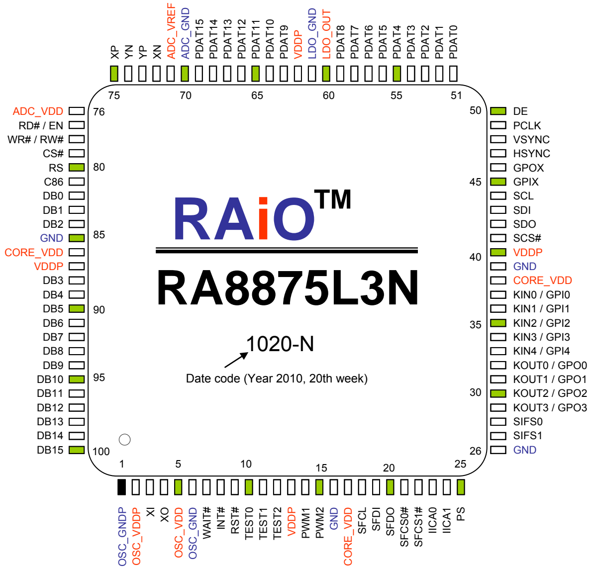
图 9-1 : RA8875 的接脚图
