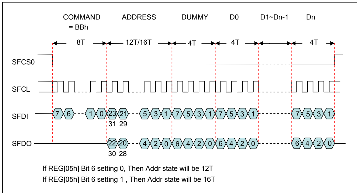
图 6-40 : 双倍模式 - 1 读取
