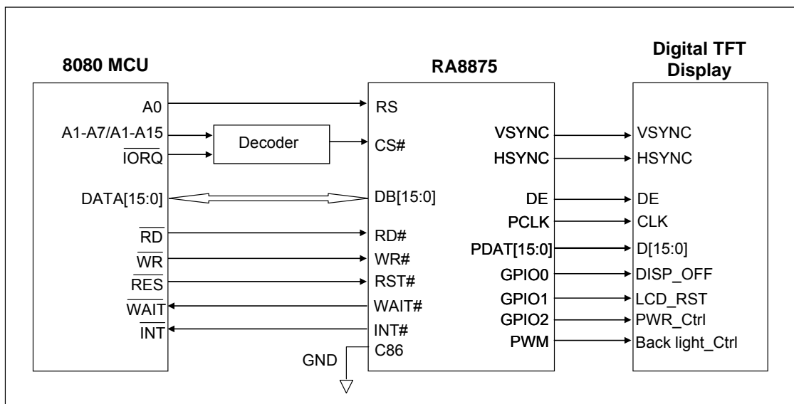
图 6-34 : RA8875 与数位 TFT 界面
