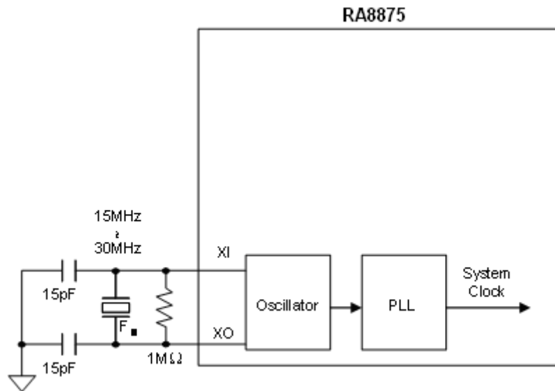
图 6-48 : 石英振荡电路与系统频率的产生
