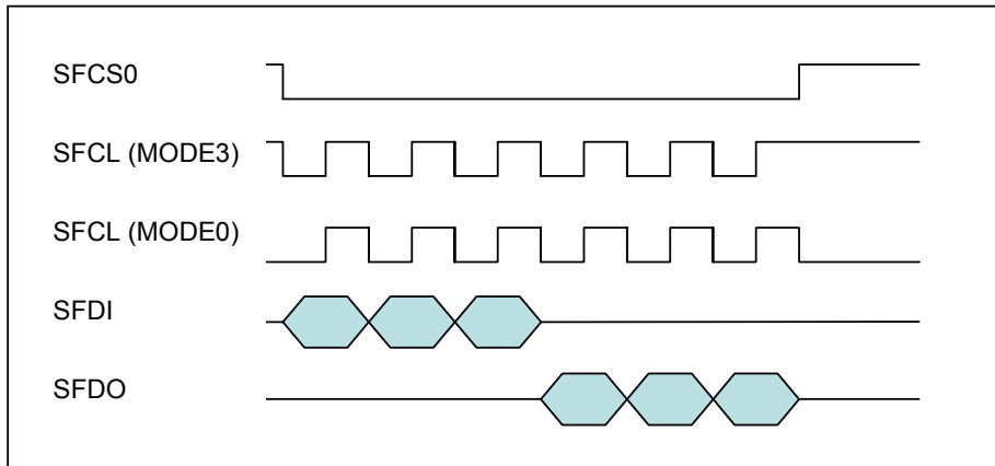
图 6-36 : Mode 0 与 Mode 3 的传输方式
