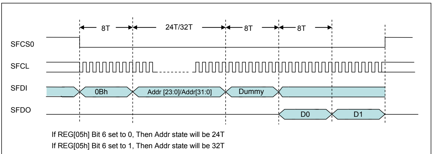
图 6-38 : 5-BUS (快速) 读取
