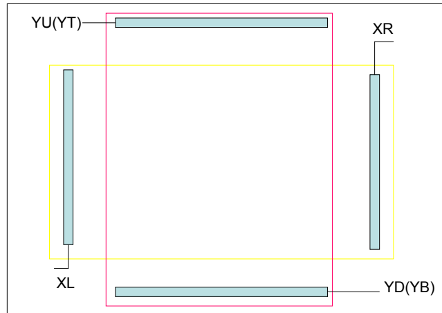
图 6-43 : 4-wire 触控面板架构
