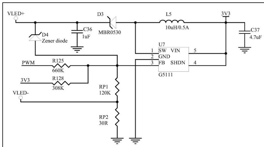
图 6-47 : PWM 控制 TFT 面板背光的应用电路
