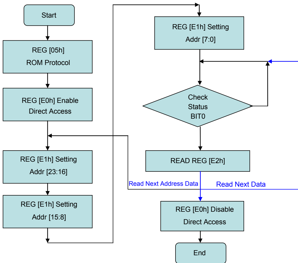
图 6-42 : 直接存取模式流程图
