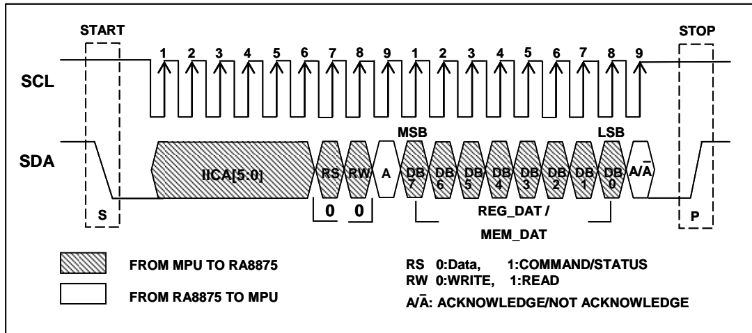
图 6-22 : IIC 数据总线的的数据写入
