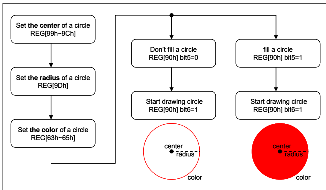
图 7-26 : 绘图功能 - 画圆
