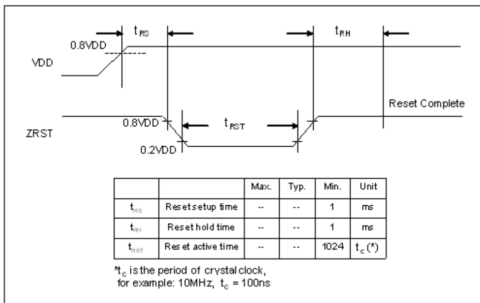
图 6-50 : 复位时序参数
