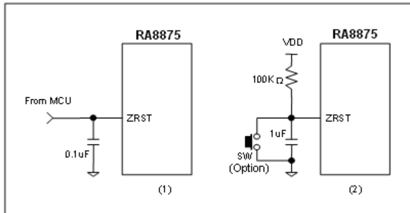
图 6-49 : RST# 接脚的使用范例
