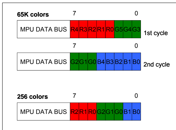
图 6-31 : MCU 8-bit 时 Data Bus 所对应到的 RGB 数据
