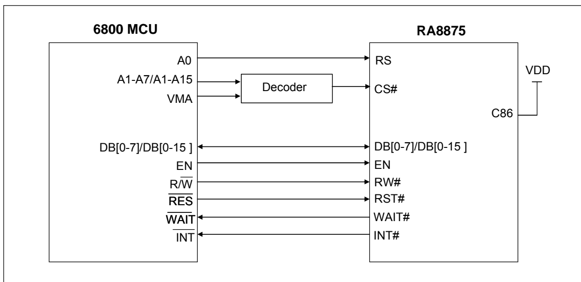
图 6-2 : 6800 MCU 界面
