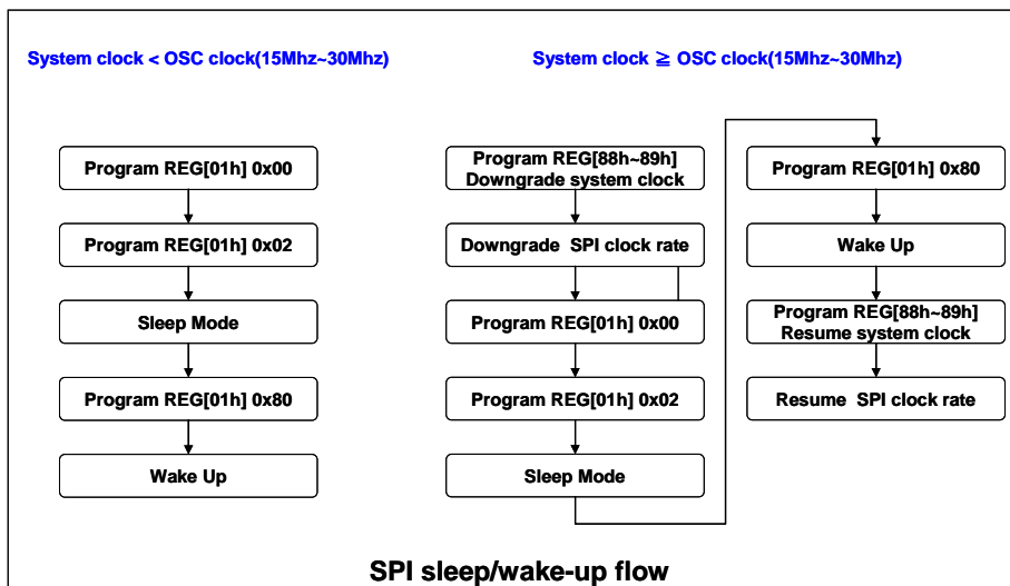
图 6-19 : SPI 睡眠/喚醒流程
