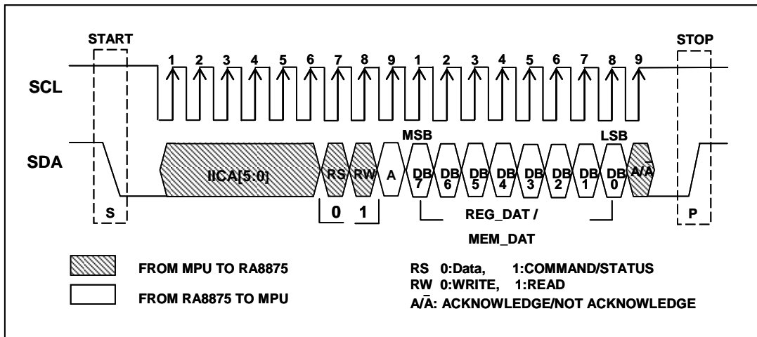
图 6-23 : IIC 数据总线的的数据读取
