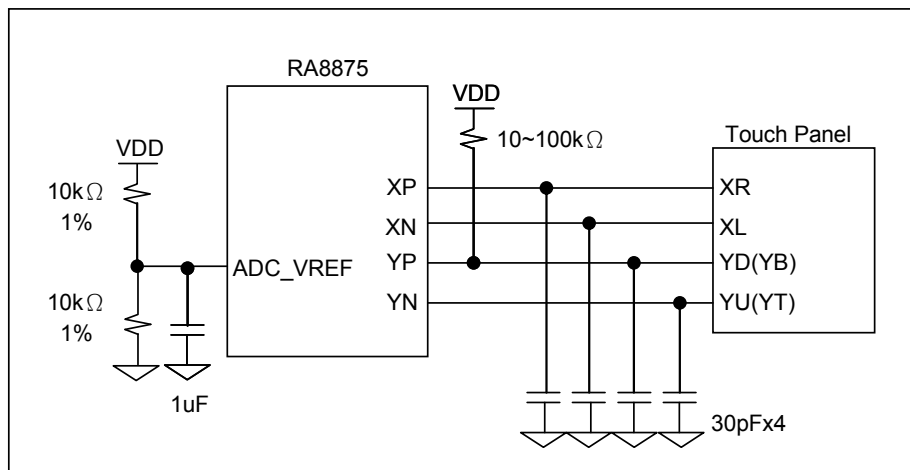
图 6-45 : 4-wire 触控面板应用电路
