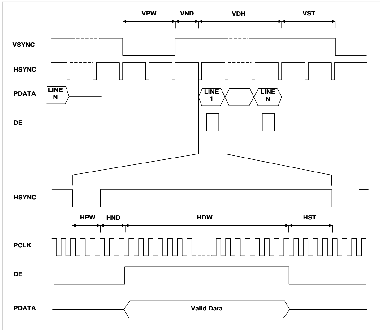
图 6-33 : 数位 TFT 面板时序图
