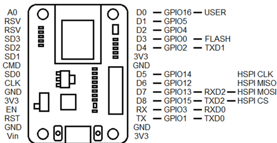
Figure 6 驱动板的引脚定义
